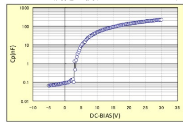
C-V測定の場合(W32-IM3536BIAS)
