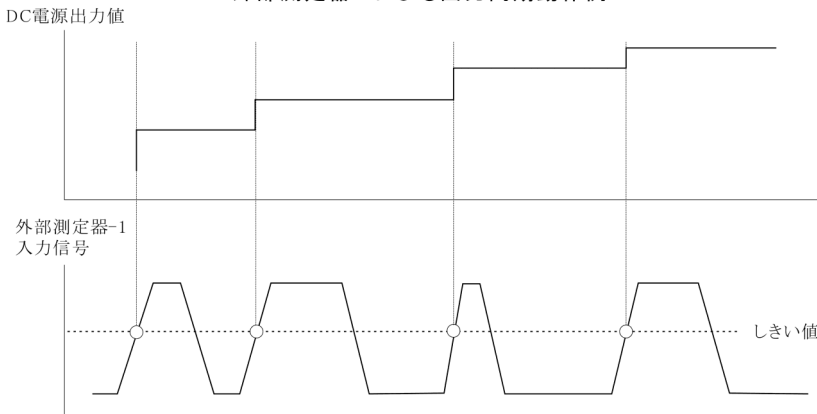
外部測定器-1による出力同期動作例
